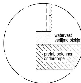
doorsnede A-A
